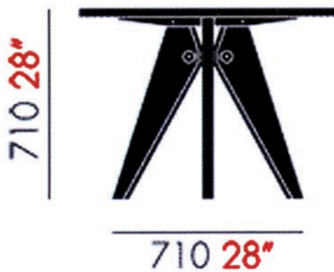
IMAXE 2: Mesa Guéridon, que Jean Prouvé deseñou en 1949 para a Universidade de París, reeditada polo Vitra Design Museum. Datos en negro: mm. Datos en vermello: polgadas.
